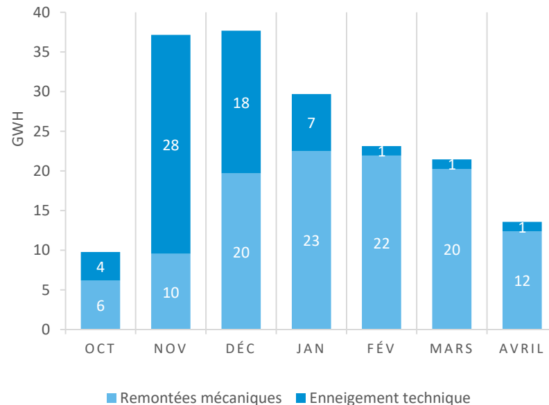
Répartition RM versus enneigement technique GWh Mois d'hiver (2021)
